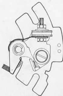
ANCIEN MODELE RUPTEUR 20914 FONCTIONNANT AVEC CAME 20927
